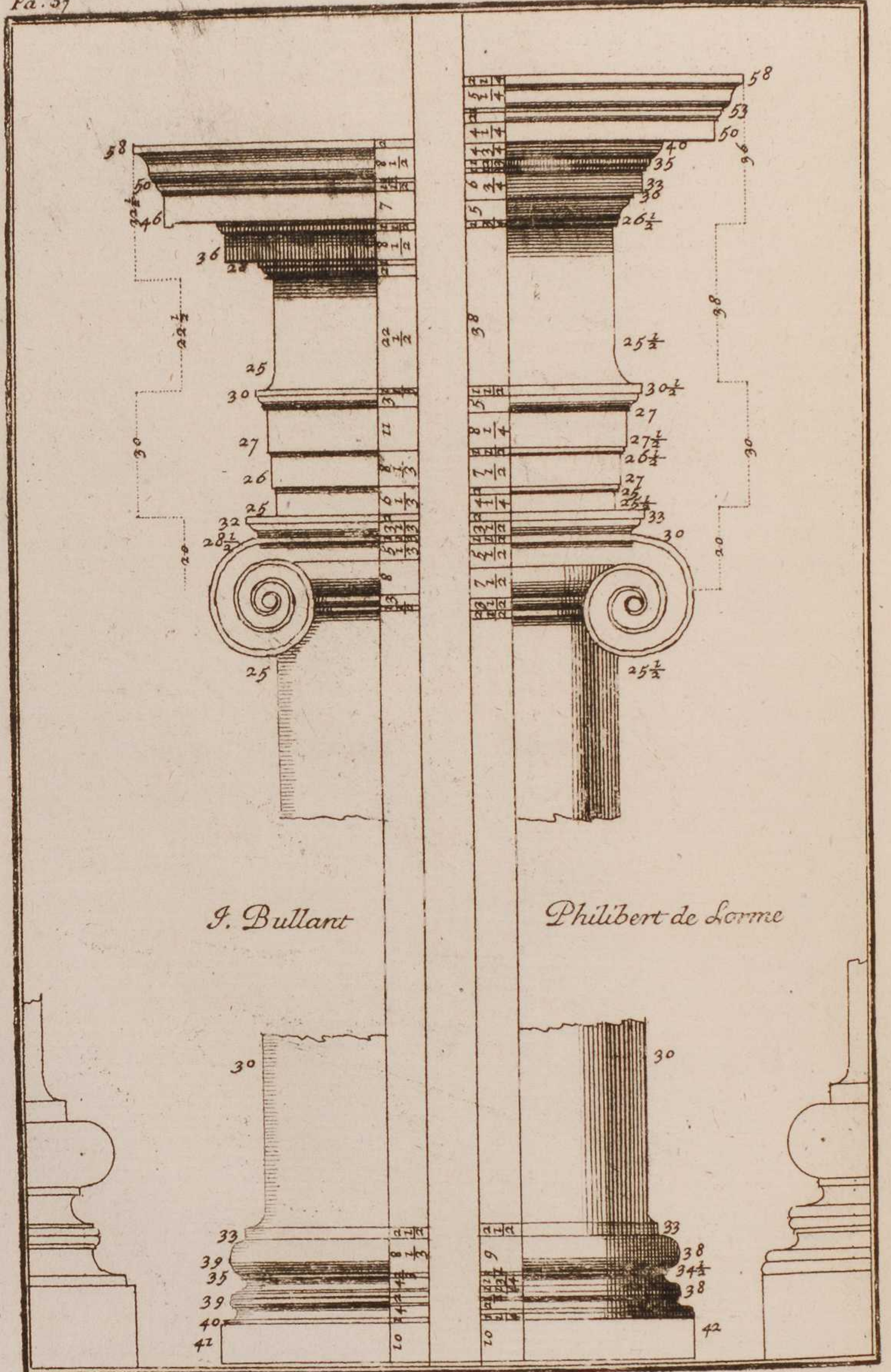
Ordre Ionique
