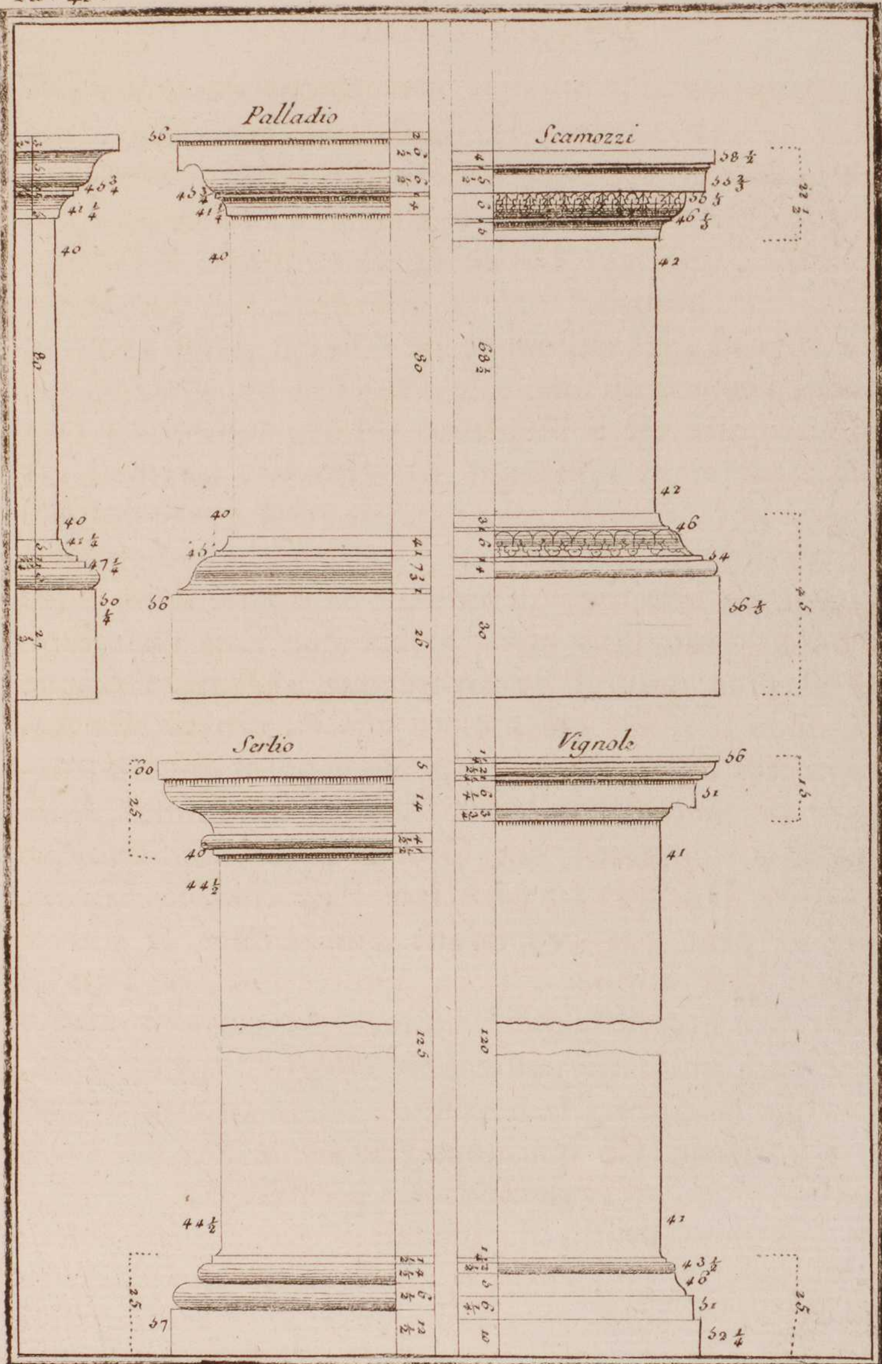
Ordre Dorique
