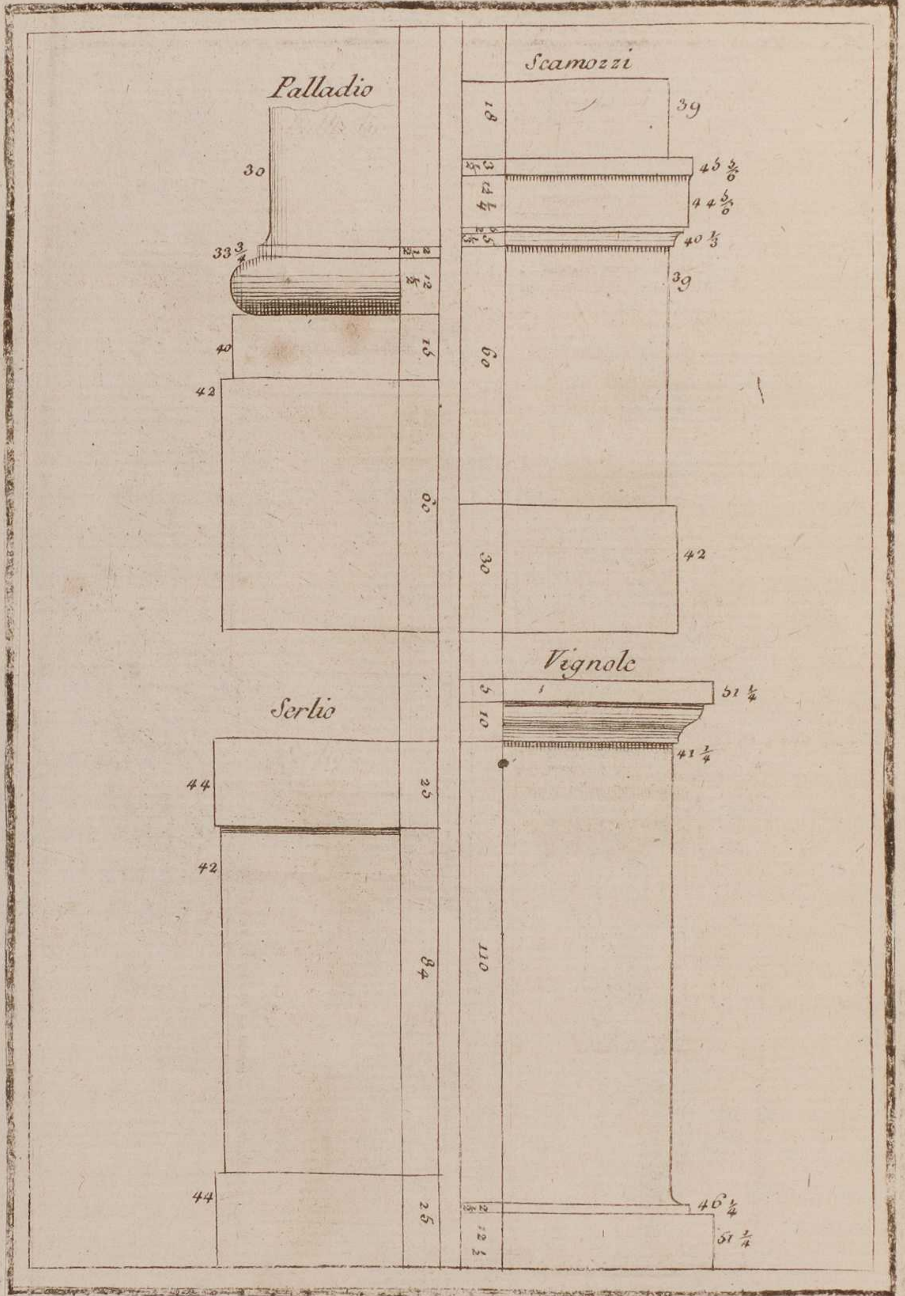
Ordre Toscan
