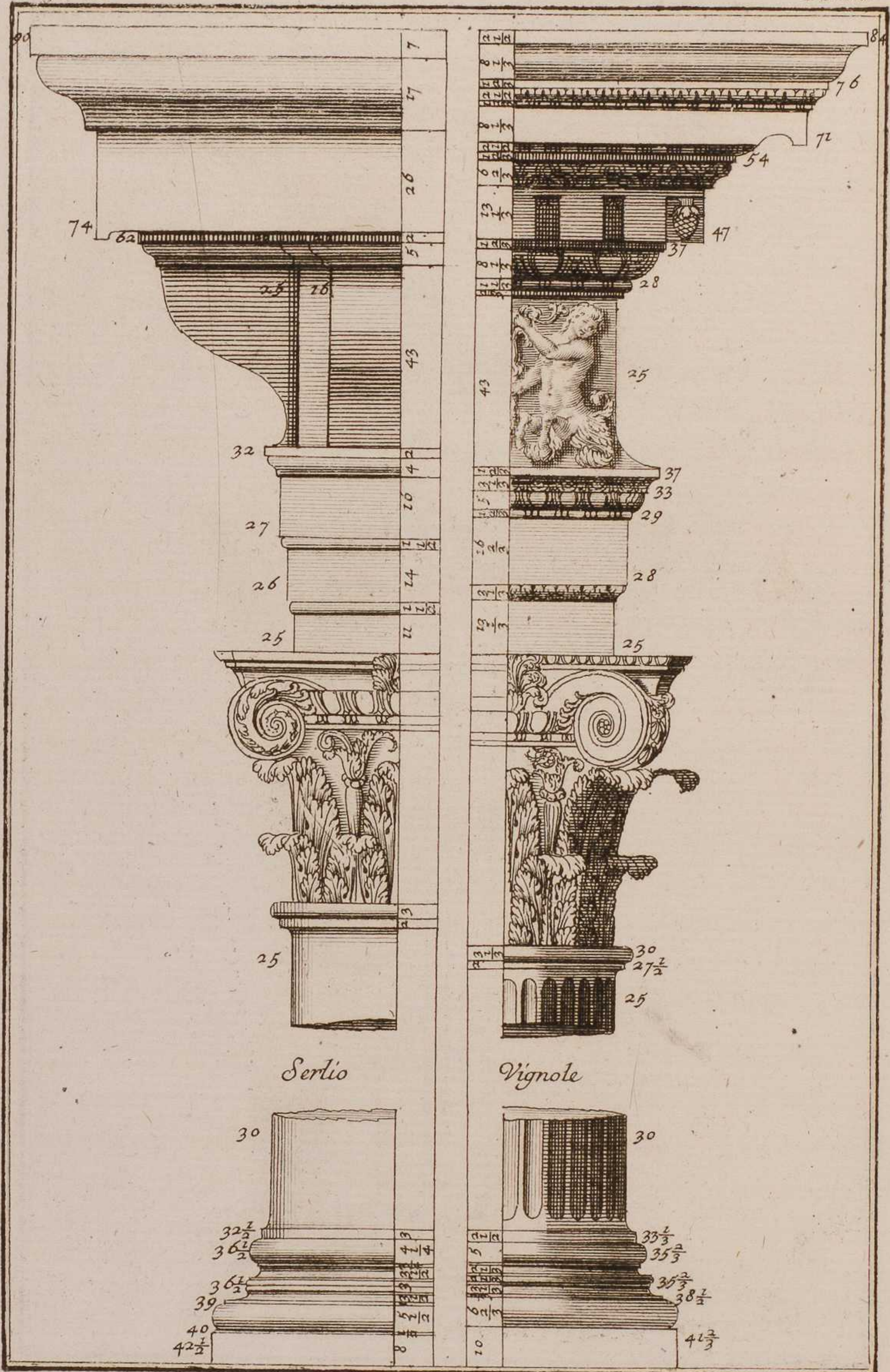
Ordre Composite
