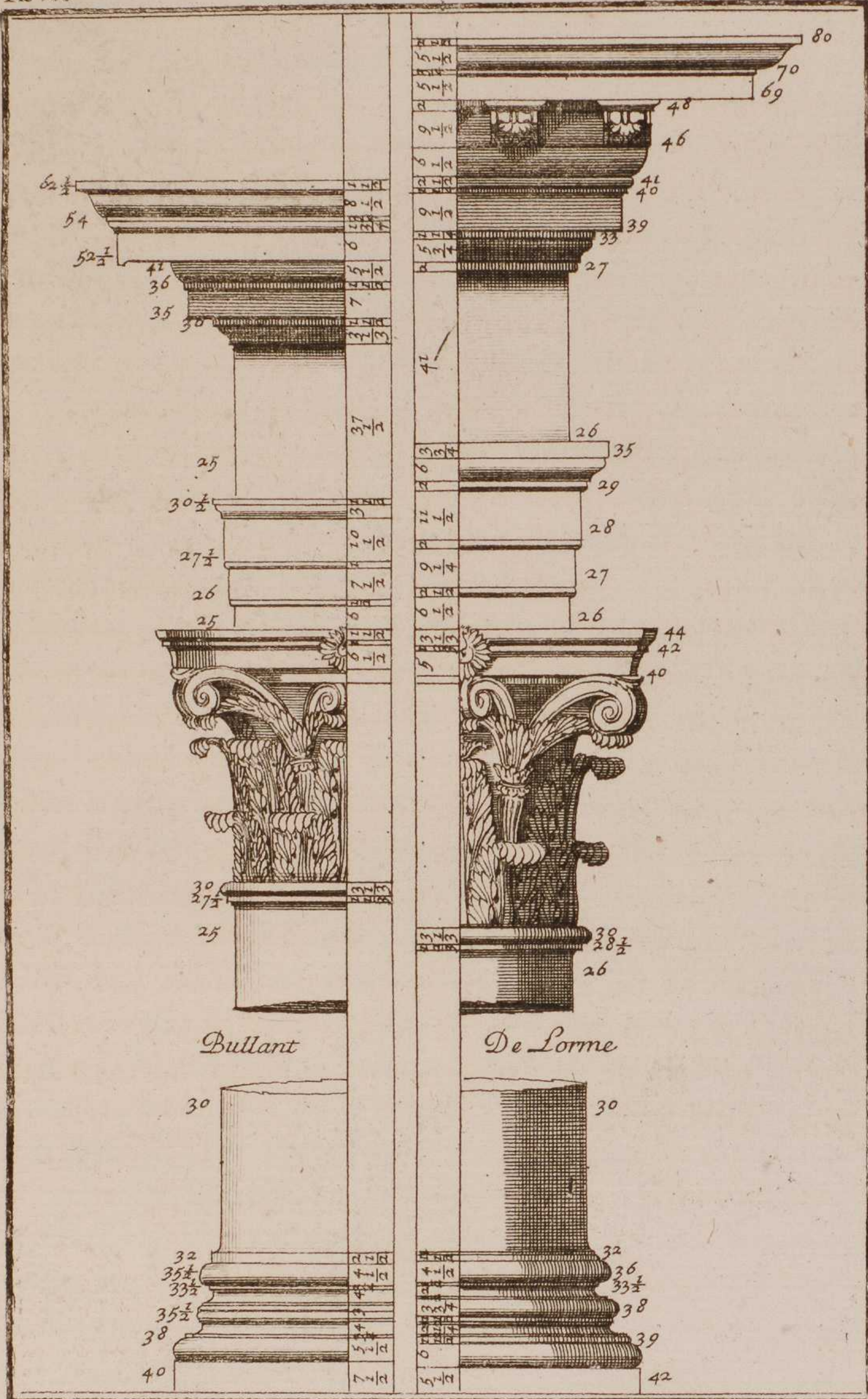
Ordre Corinthien
