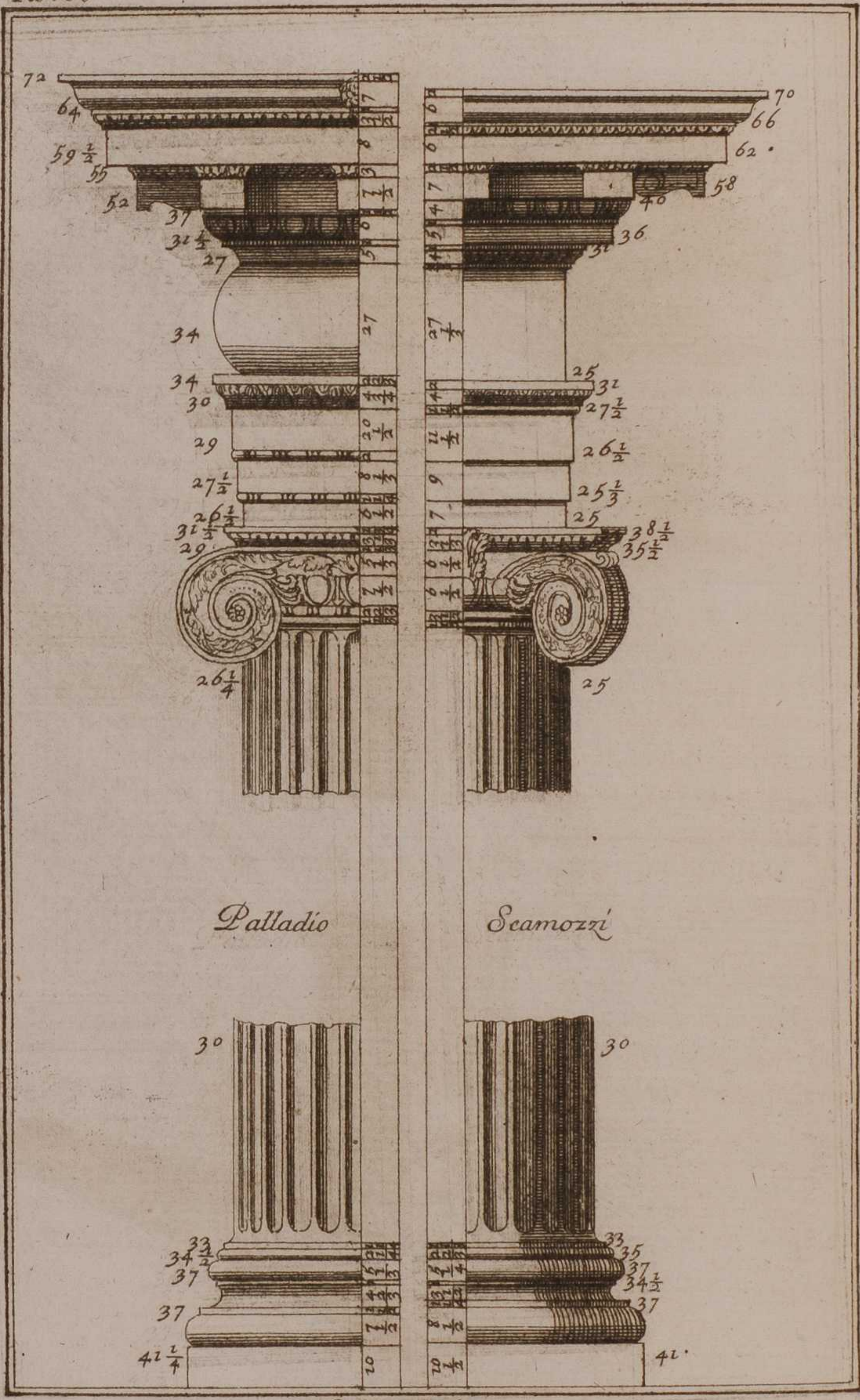
Ordre Ionique
