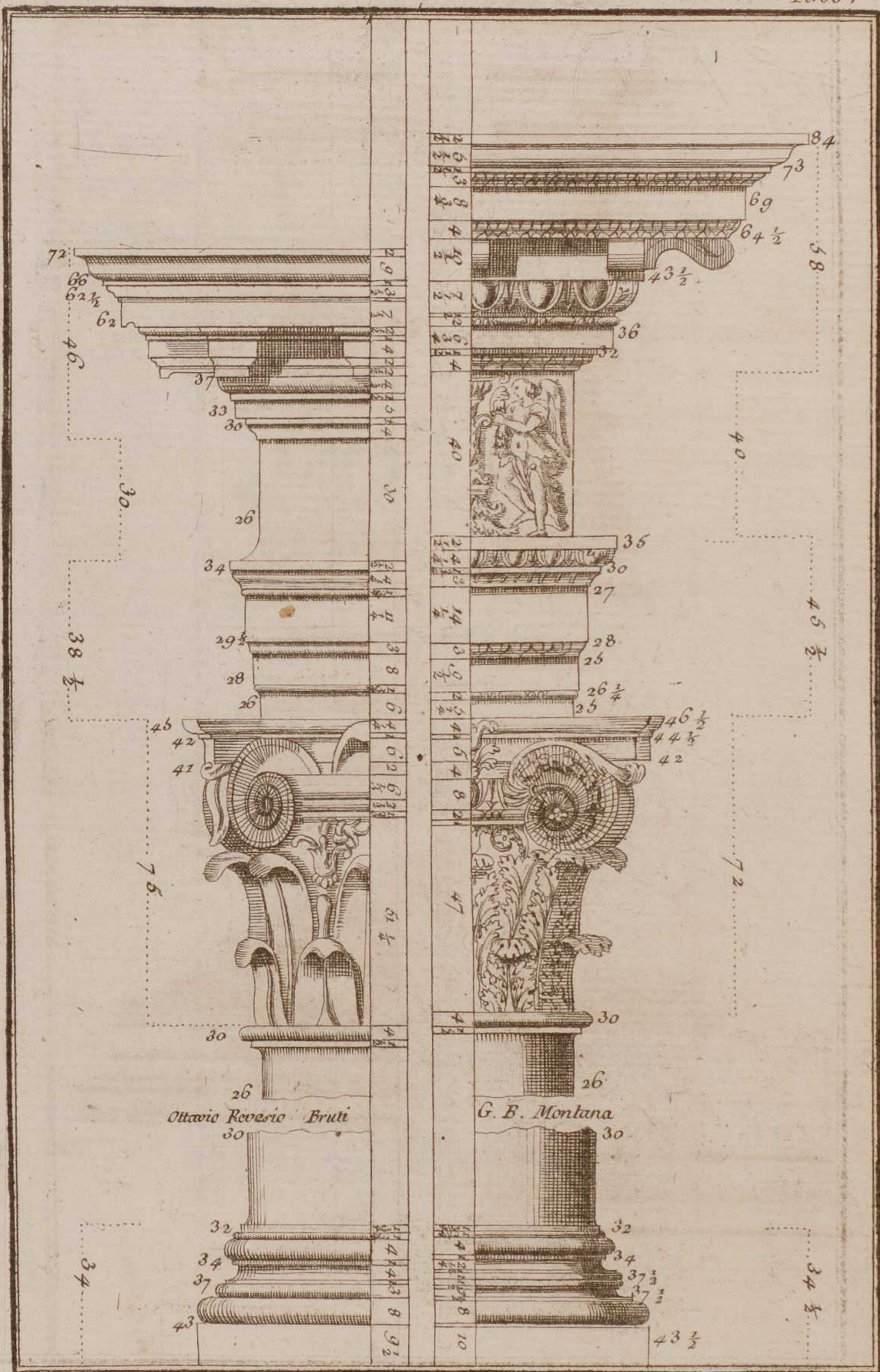
Ordre Composite
