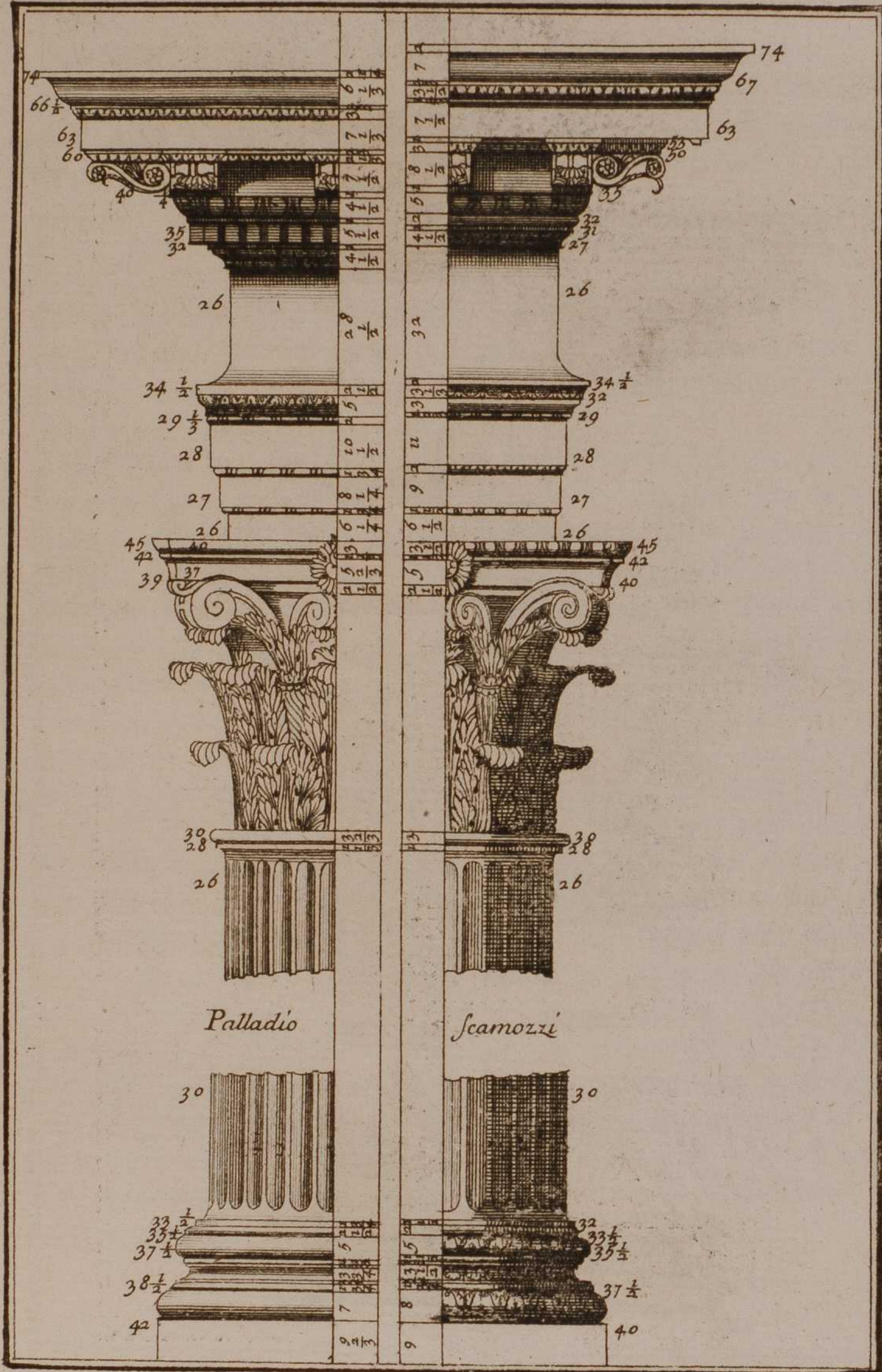
ordre Corinthien
