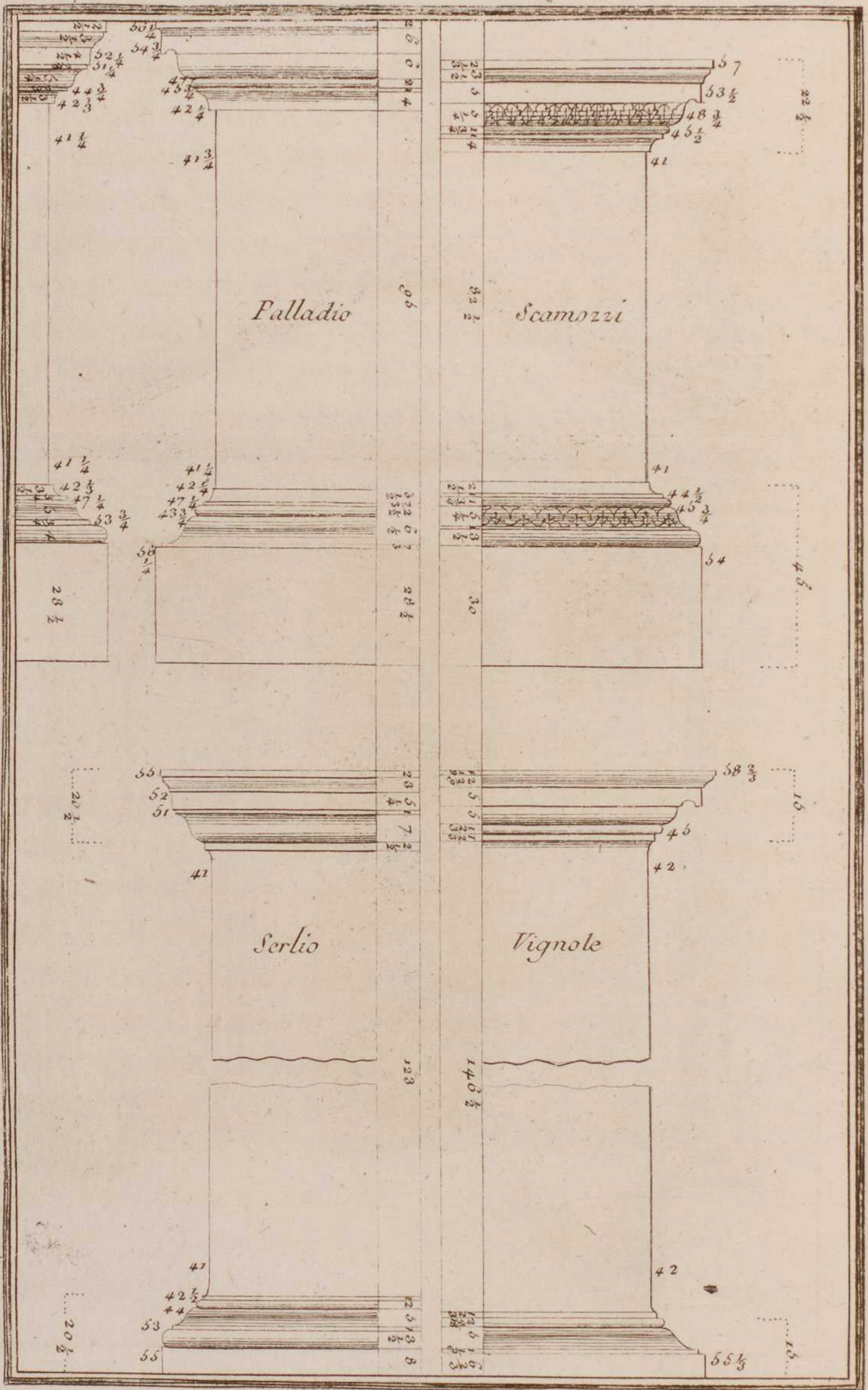
Ordre Ionique
