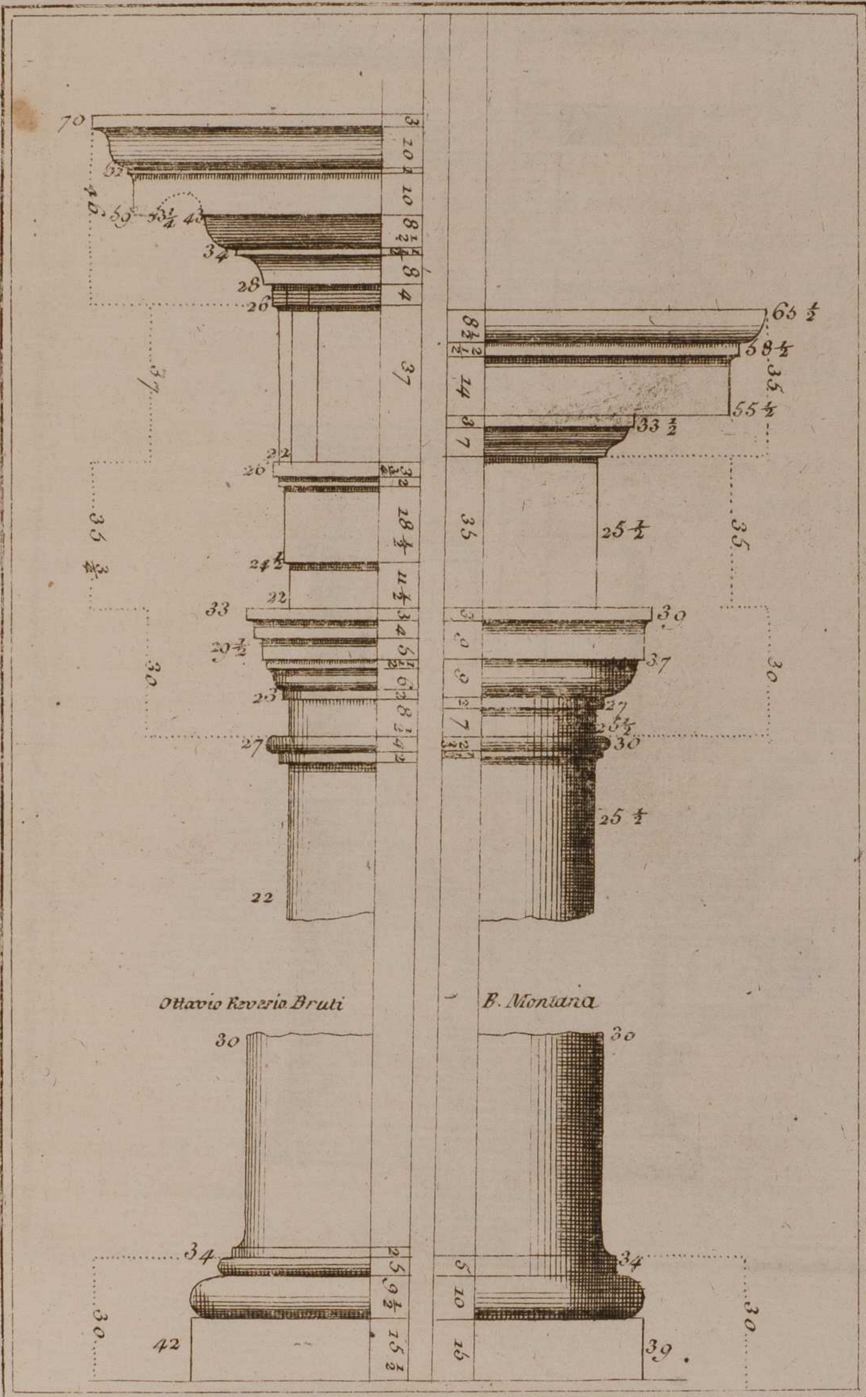
Ordre Toscan
