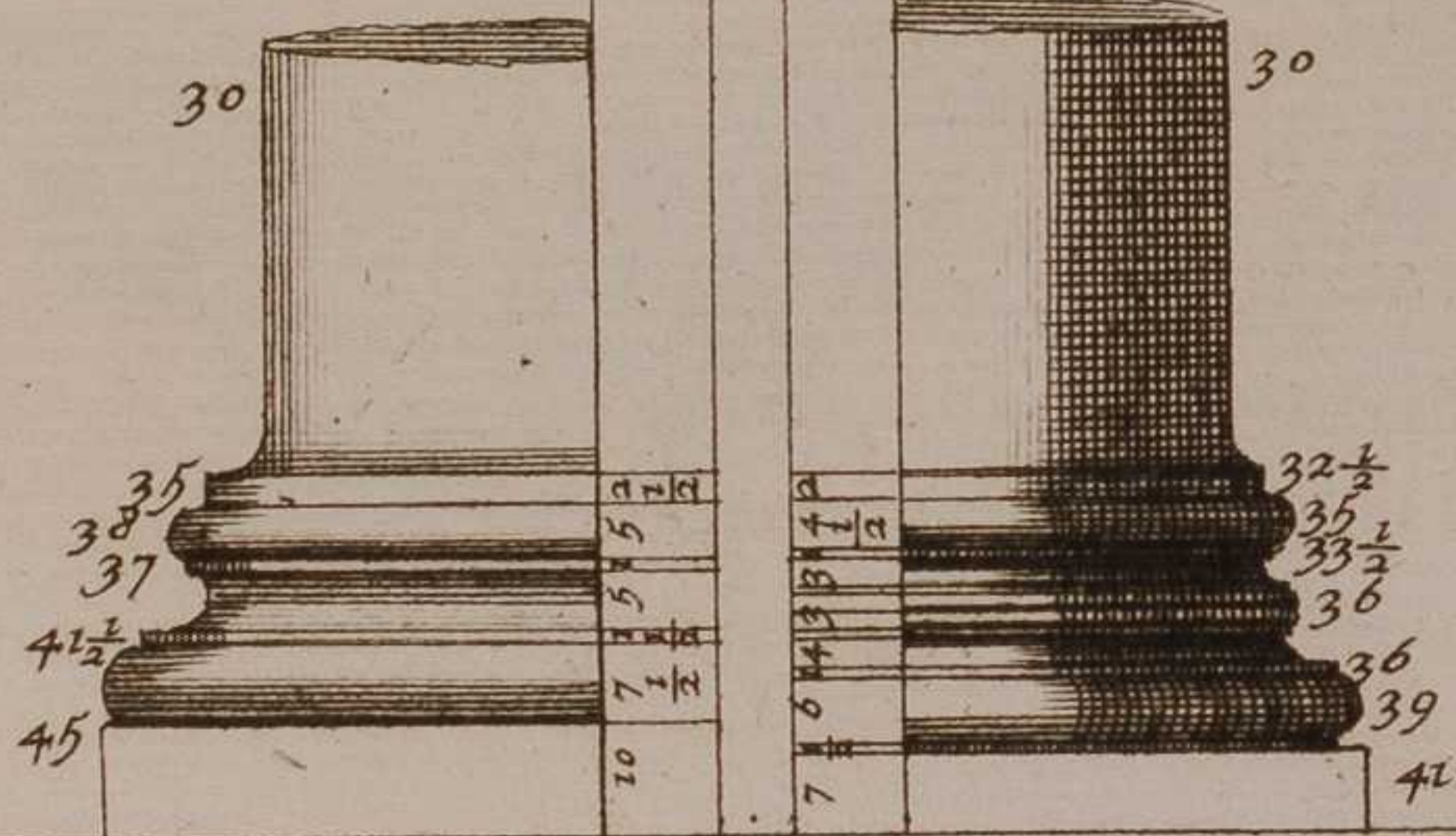
Ordre Corinthien
