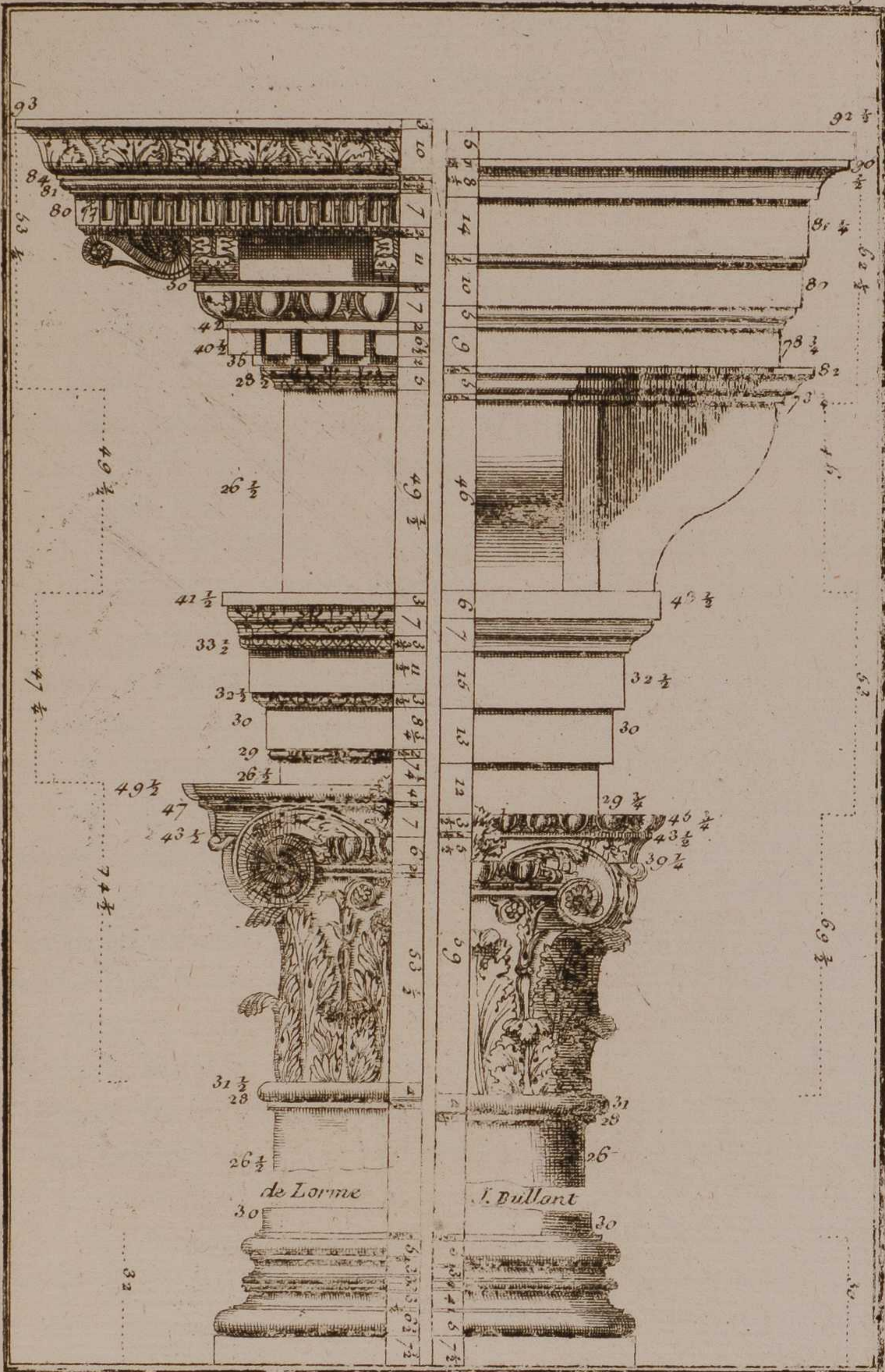
Ordre Composite
