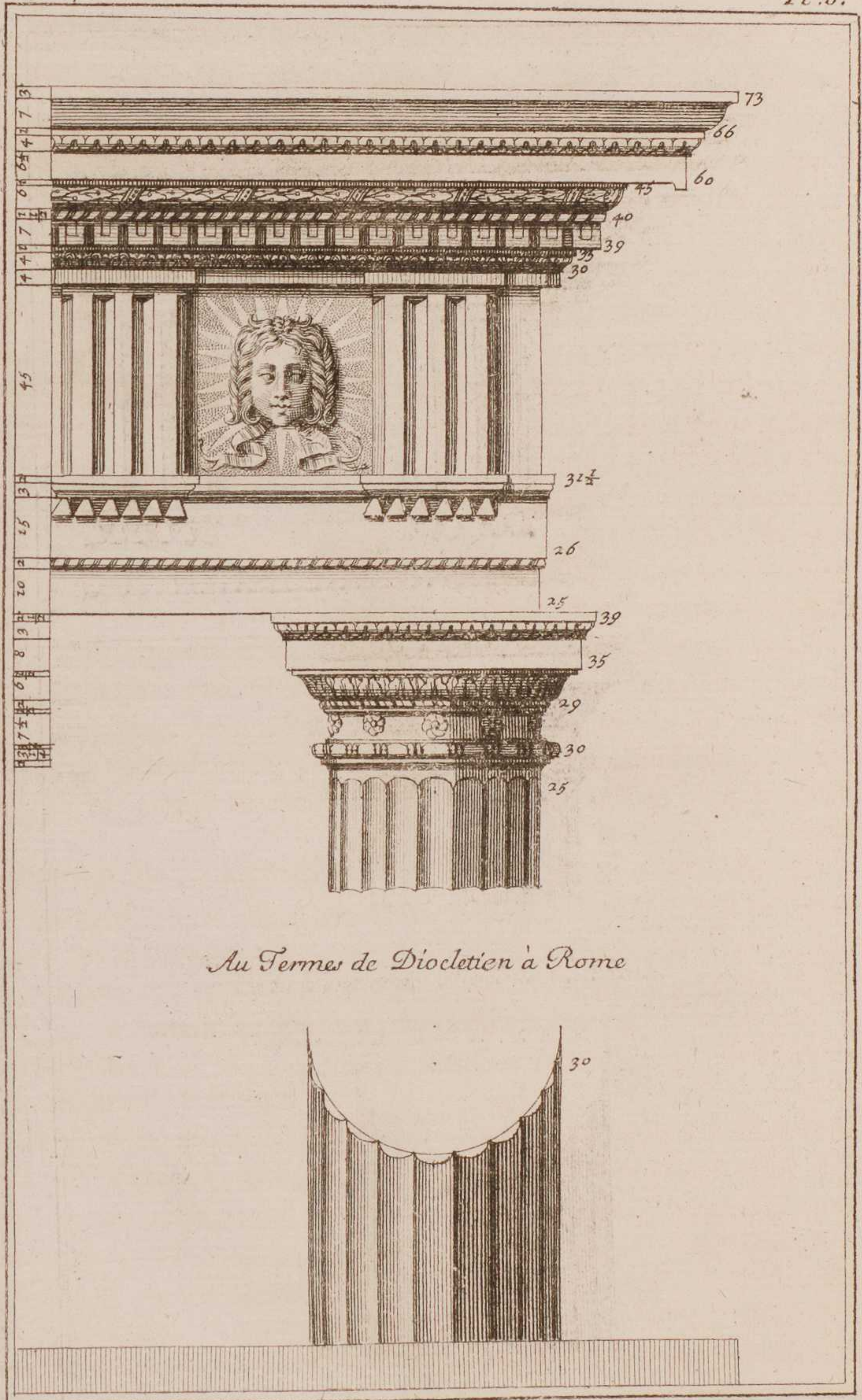
Ordre Dorique
