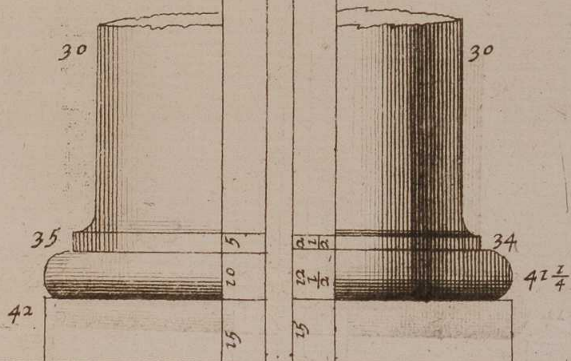
Ordre Toscan
